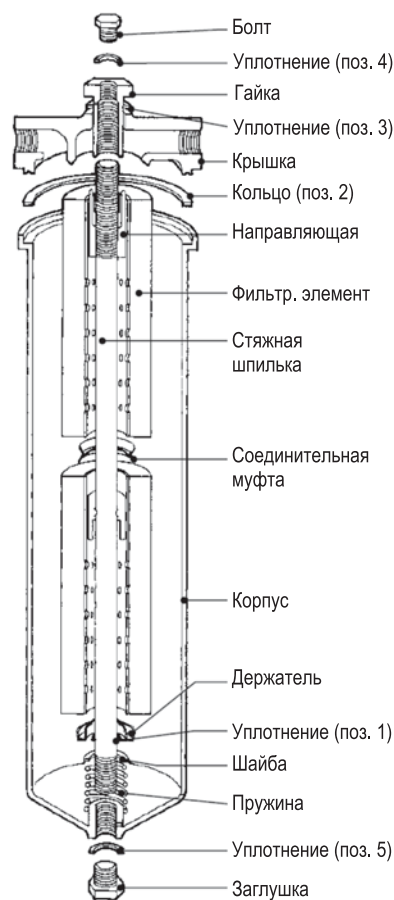
Уплотнения
