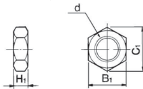
Гайка поршневого штока Материал: углеродная сталь
