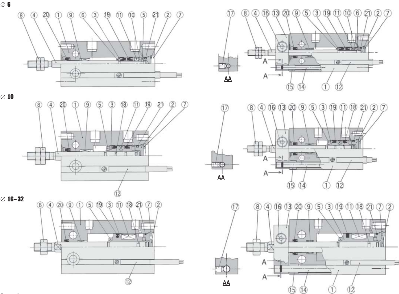
Цилиндр CDUK с защитой от проворота штока
