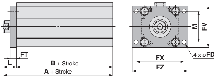
Rod Flange
