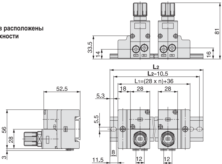
ARM11BC2 Ручки регуляторов расположены снизу
